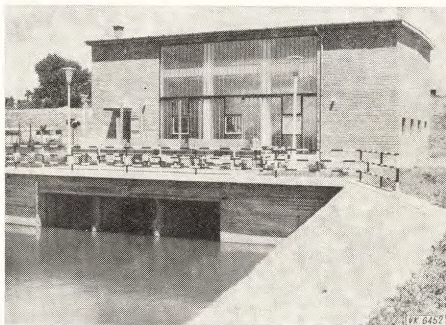
4. ábra. Nagyzugi 6 \text{ m}^3/\text{sec} teljesítményű belvízátemelő szivattyútelep
