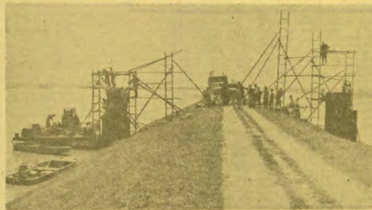
A Fehér-Körös töltésén épült a képen látható állványzat. A gyulai ÁKSZ dolgozói a visszaramló víz további pusztításától védik a gátat.
