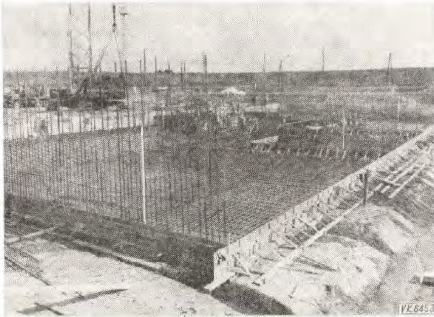
5. ábra. A Körösladányi Duzzasztómű építése a Sebes-Körösön
