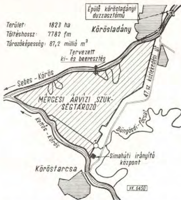
2. ábra. Mérgesi árvízi szükségtározó helyszínrajza
