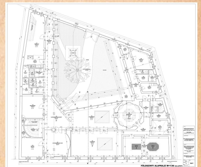
Megvalósult állapotterv, földszinti alaprajz 2011
